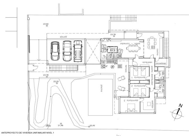
ANTEPROYECTO DE VIVIENDA UNIFAMILIAR NIVEL 1
